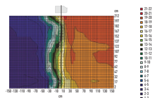
Ouverture avec un rideau d'air correctement adapté.
