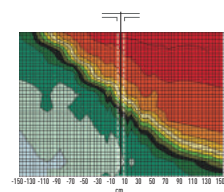
Ouverture sans rideau d'air.
