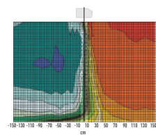
Ouverture avec rideau d'air, vitesse trop élevée.
