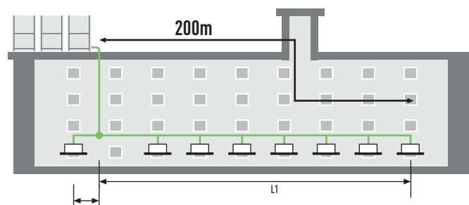
L1 = Tuyauterie la plus longue. L2 = Tuyauterie la plus courte. L1 - L2 = 50 m maximum
